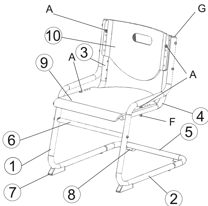
Вид спереди
